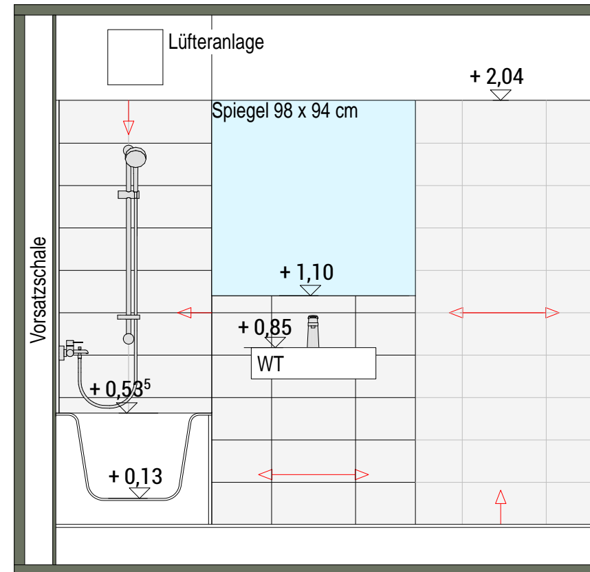
Ansicht 4
