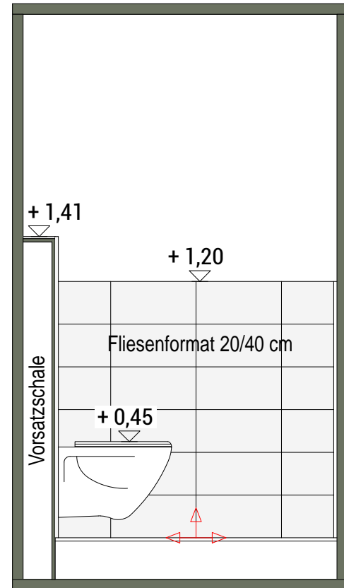
Ansicht 1
