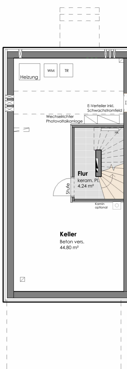
KELLERGESCHOSS
