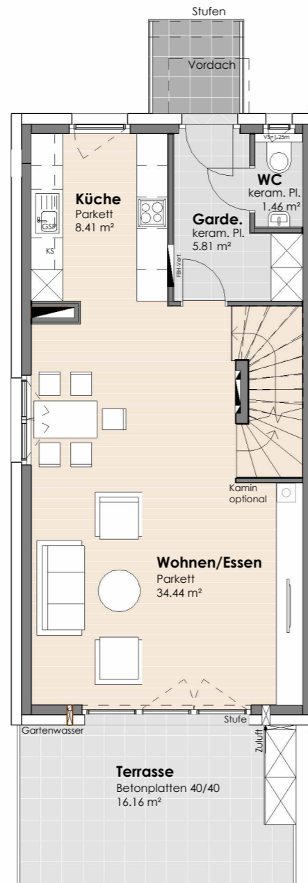
ERDGESCHOSS
