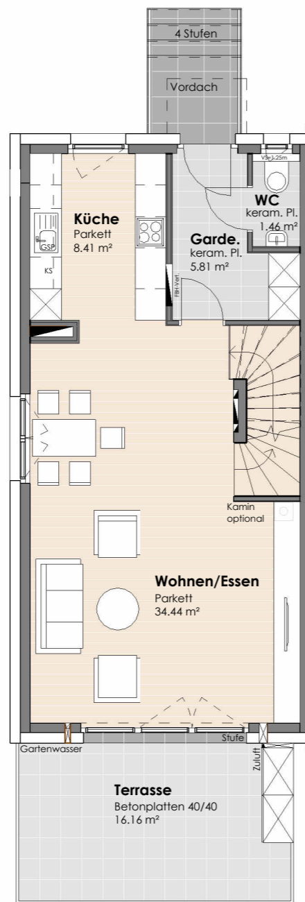
ERDGESCHOSS
