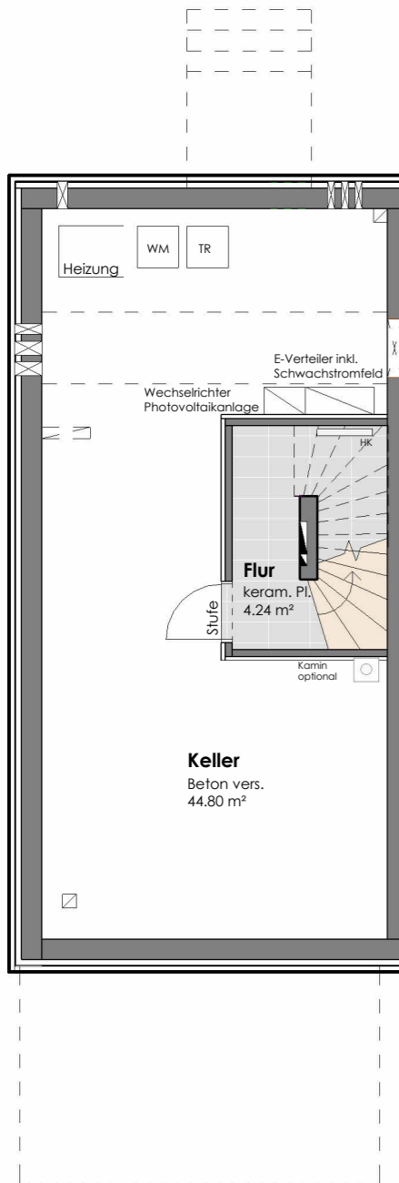
KELLERGESCHOSS
