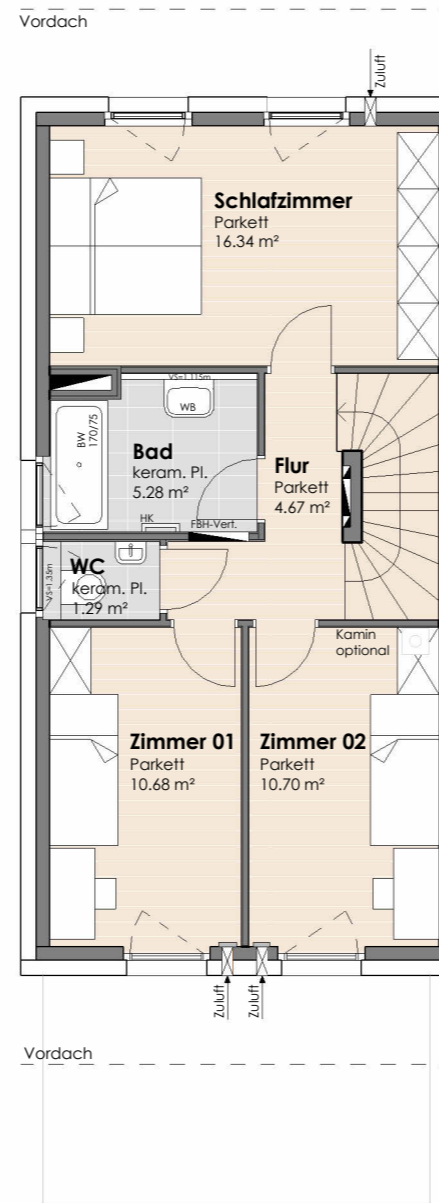
OBERGESCHOSS
