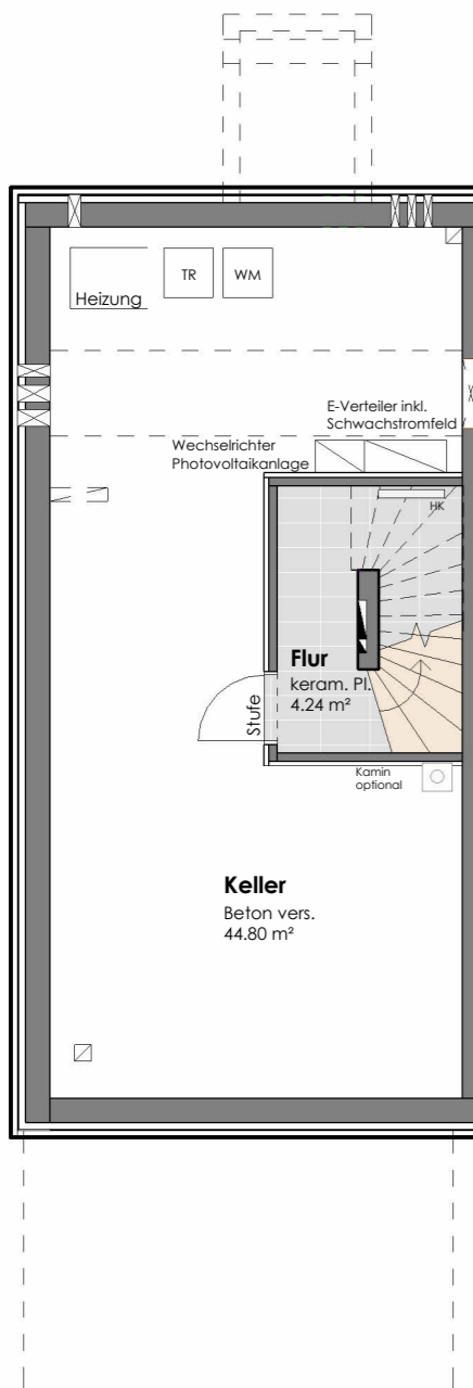
KELLERGESCHOSS
