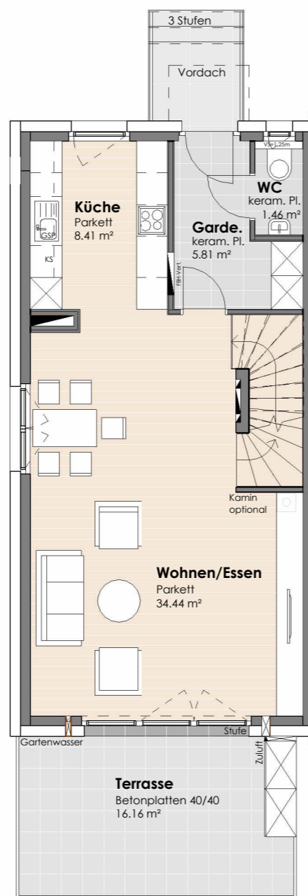
ERDGESCHOSS
