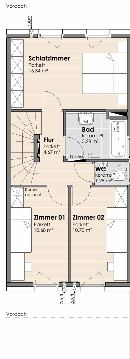
OBERGESCHOSS
