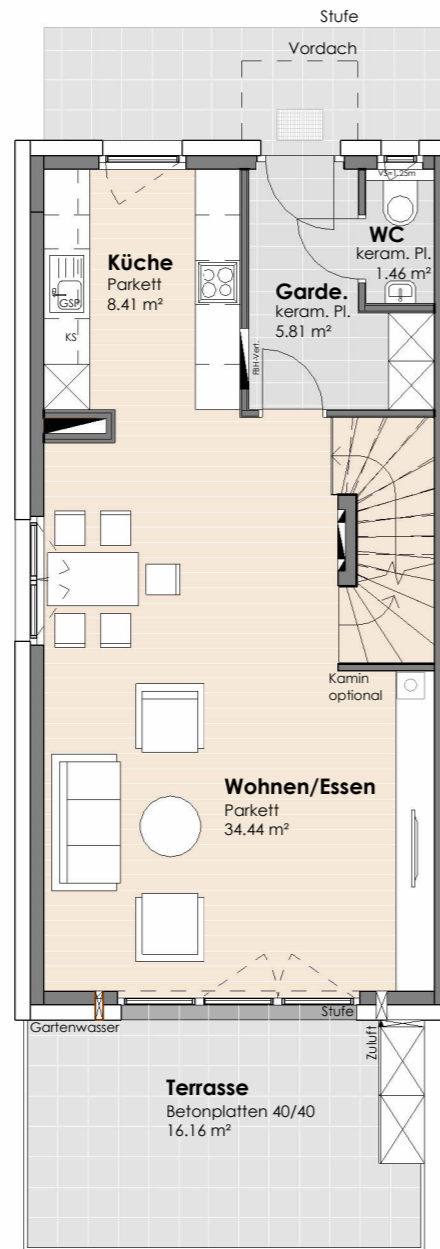
ERDGESCHOSS
