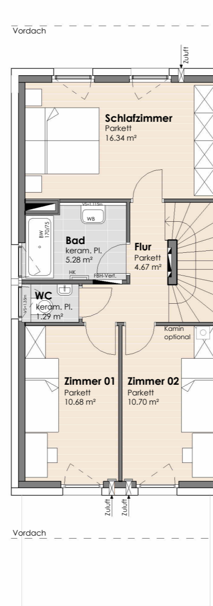
OBERGESCHOSS
