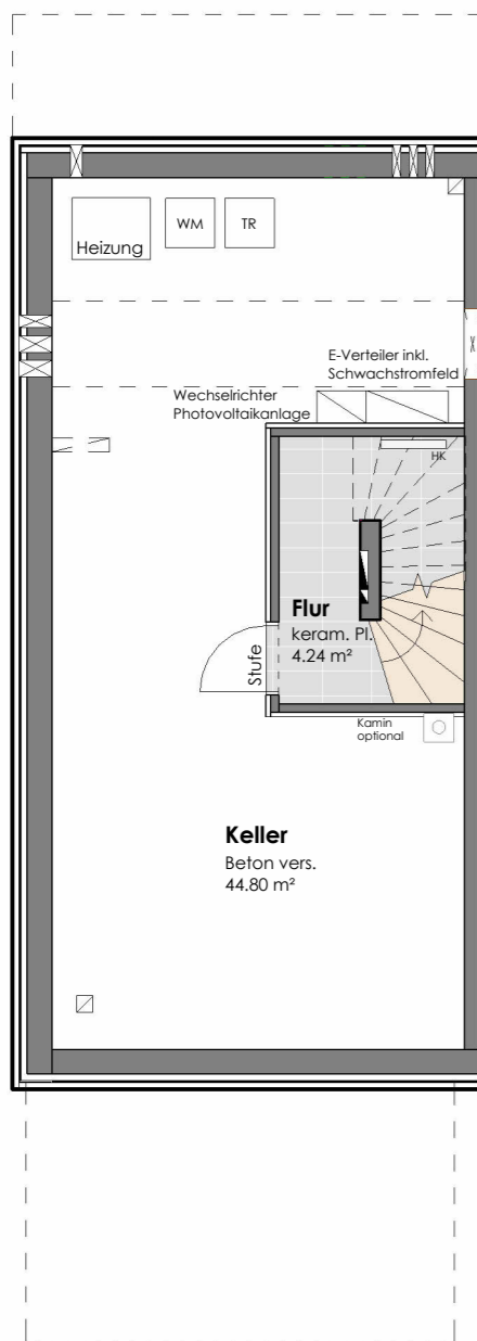
KELLERGESCHOSS
