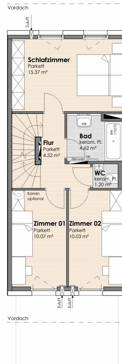
OBERGESCHOSS
