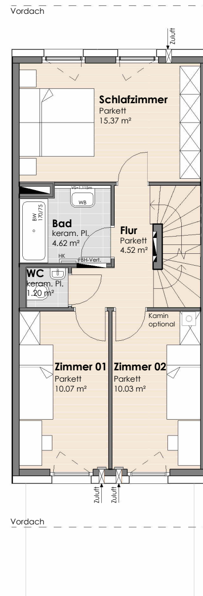
OBERGESCHOSS
