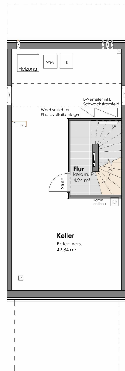
KELLERGESCHOSS
