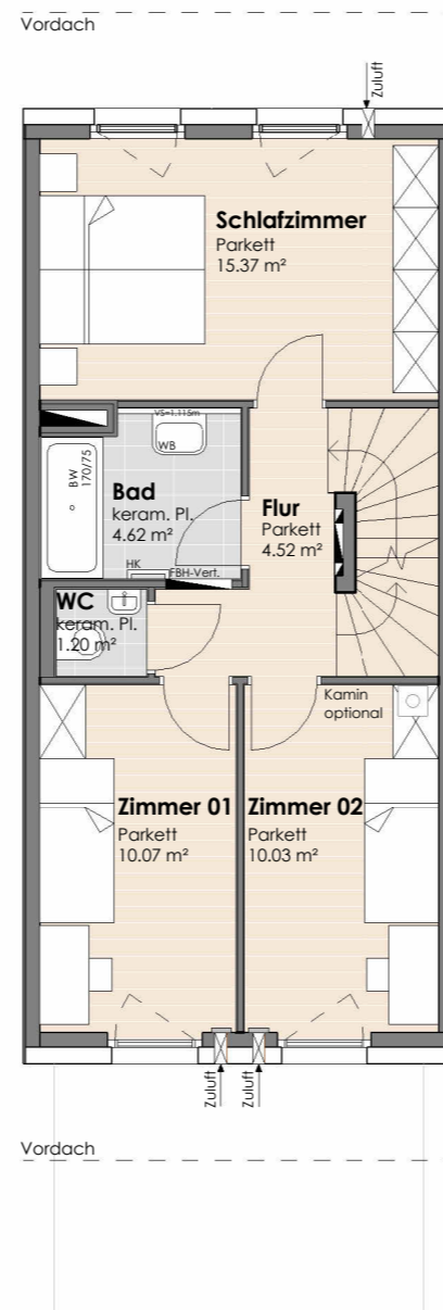
OBERGESCHOSS
