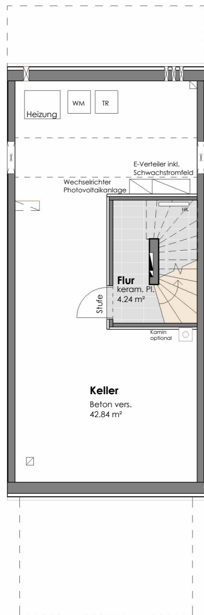
KELLERGESCHOSS
